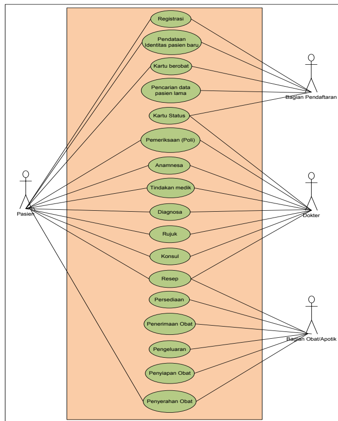
Gambar 4.17 Use Case Diagram Detail Pelayanan Kesehatan Puskesmas
