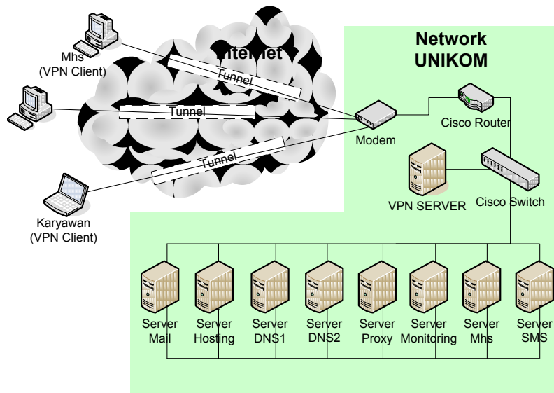
Gambar 3. Arsitektur VPN Unikom
