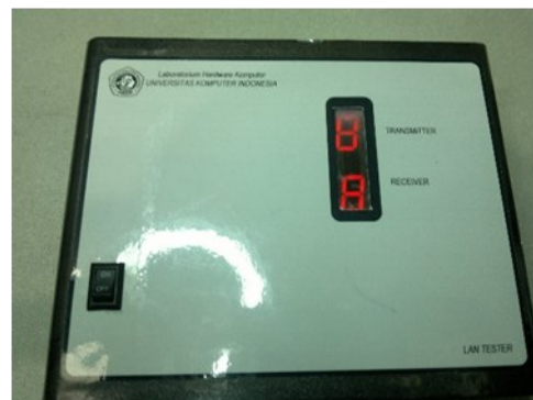
Gambar 12. Desain LAN Tester yang telah selesai dirakit tampak atas
